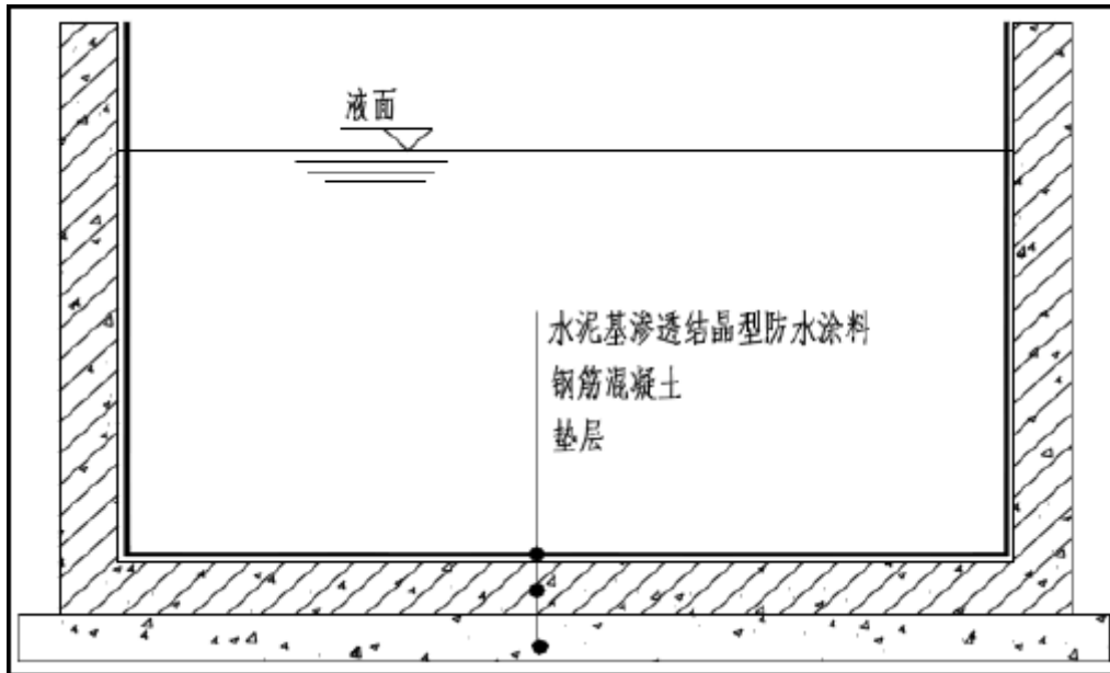
图 7-5-1 重点污染防治区水池防渗示意图
