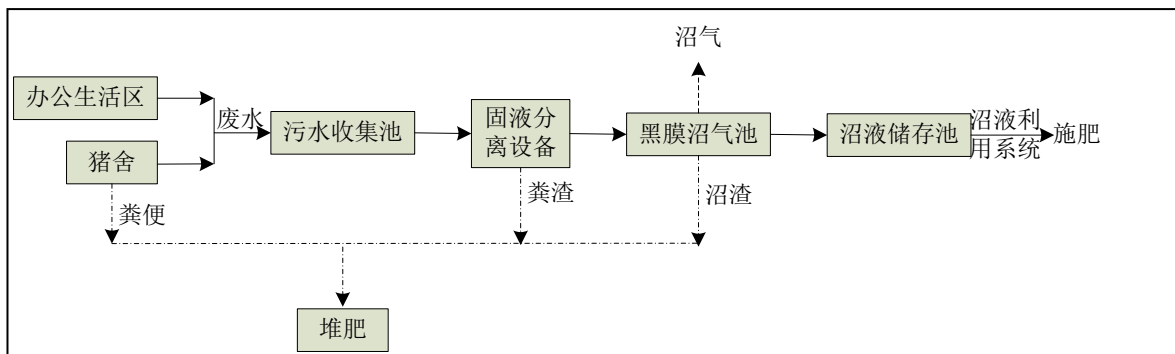
图7-3-1 项目污水处理工艺流程图
