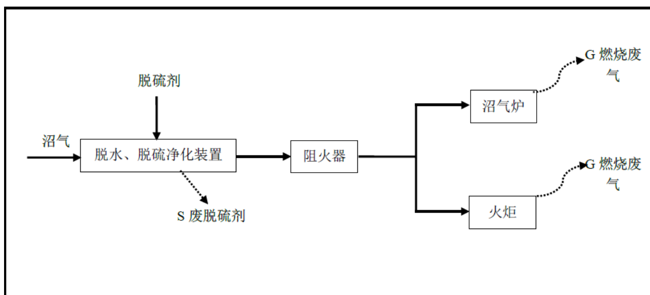
图 3-2-10 沼气利用及产污节点图
