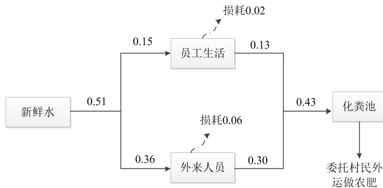
图 2-1 项目日水平衡图 (m 3 /d)
